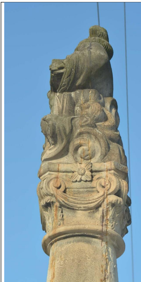
ROZSTÁNÍ - SOUSOŠÍ NEJSVĚTĚJŠÍ TROJICE, parc.číslo 169/2 TRHLINY V HLAVICI A DŘÍKU SLOUPU
